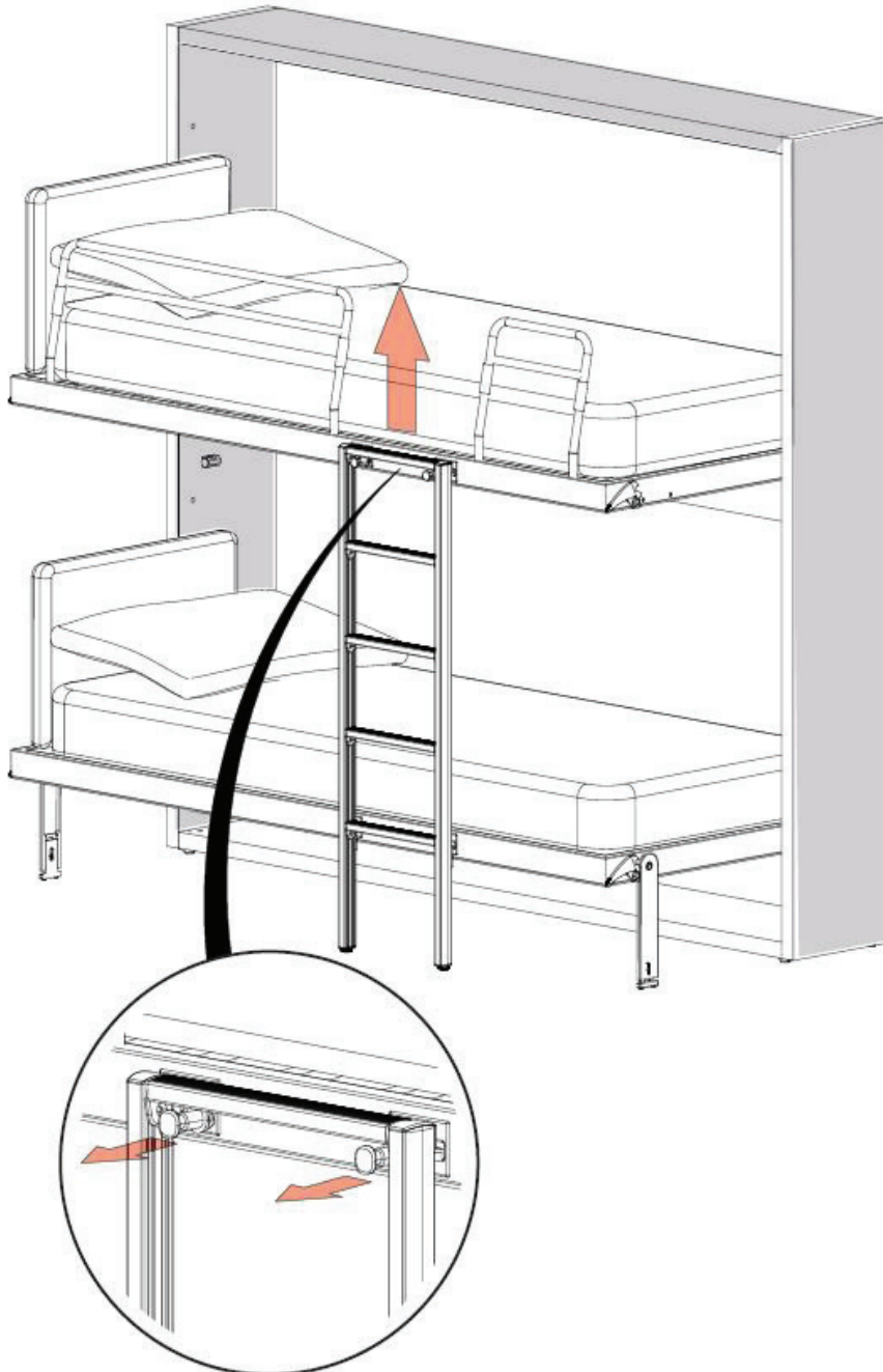
dett. 25a
